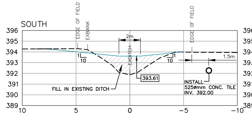
0+288 SECTION A - A
